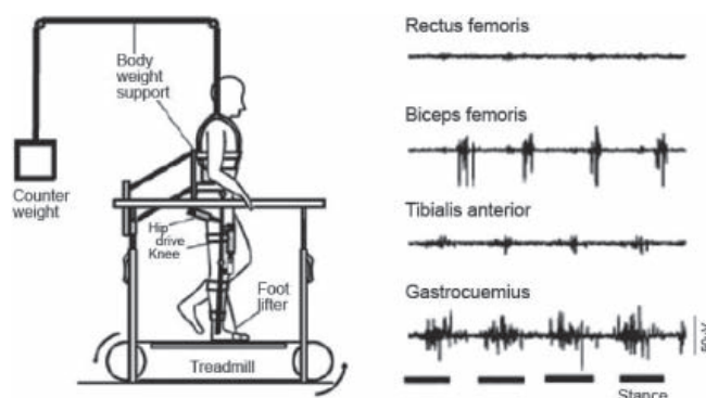
図4 脊髄損傷者を対象として脊髄CPGの特性を検討したVolker Dietzのグループの研究
