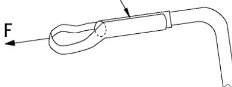
図 21 ISO7176-8 グリップ耐離脱性試験
